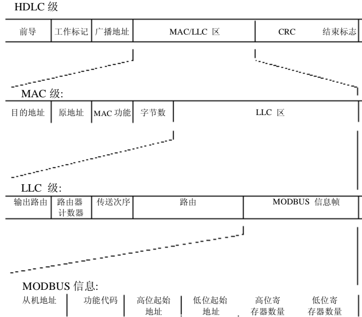
图 9: Modbus+数据内容
